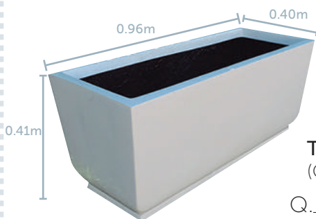
Alto 0.41m Largo 0.96m Ancho 0.40m
