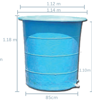
Strong 750 Capacidad para 750 litros 1.18 mt de alto 1.12 mt de diámetro
