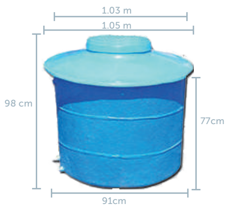
Strong 500 Capacidad para 500 litros 98cm de alto 1.03mt de diámetro
